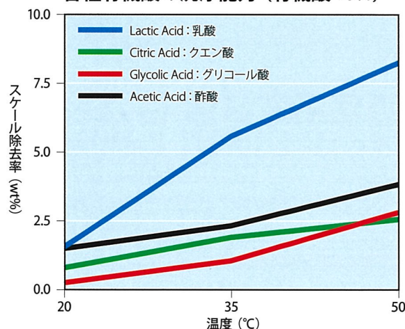
各種有機酸の洗浄能力 (有機酸 10%)
