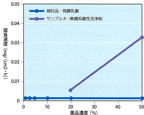
SUS304 に対する腐食速度
